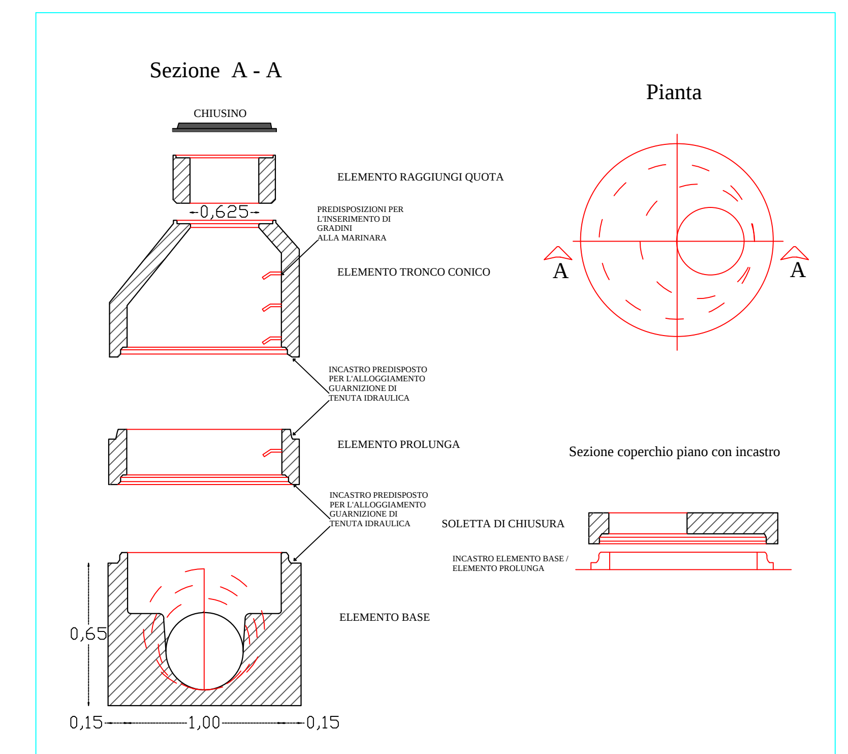
Particolari costruttivi Scala 1 : 25
