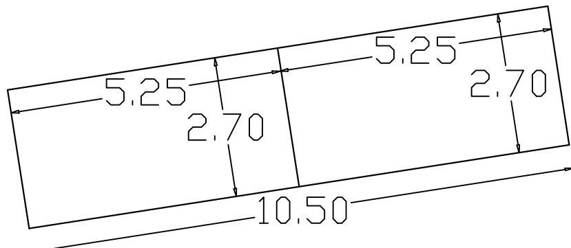
Particolare stallo autovetture
