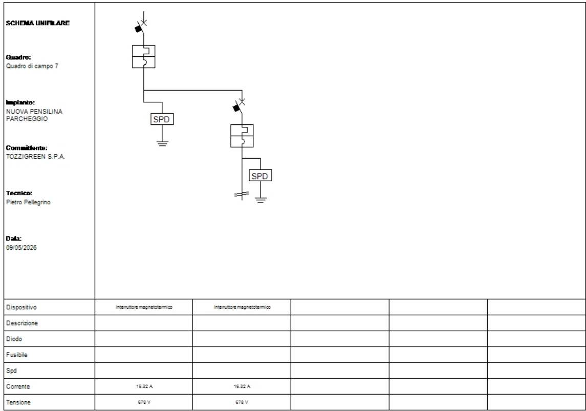
Fig. 13: Schema unifilare quadro "Quadro di campo 7"
