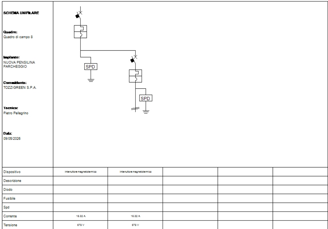
Fig. 14: Schema unifilare quadro "Quadro di campo 8"
