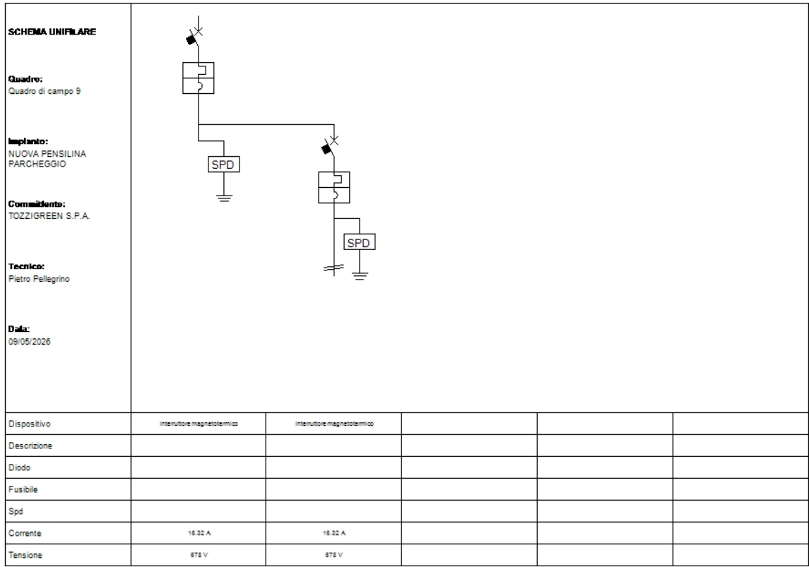
Fig. 15: Schema unifilare quadro "Quadro di campo 9"
