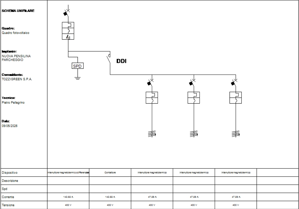
Fig. 6: Schema unifilare quadro "Quadro fotovoltaico"
