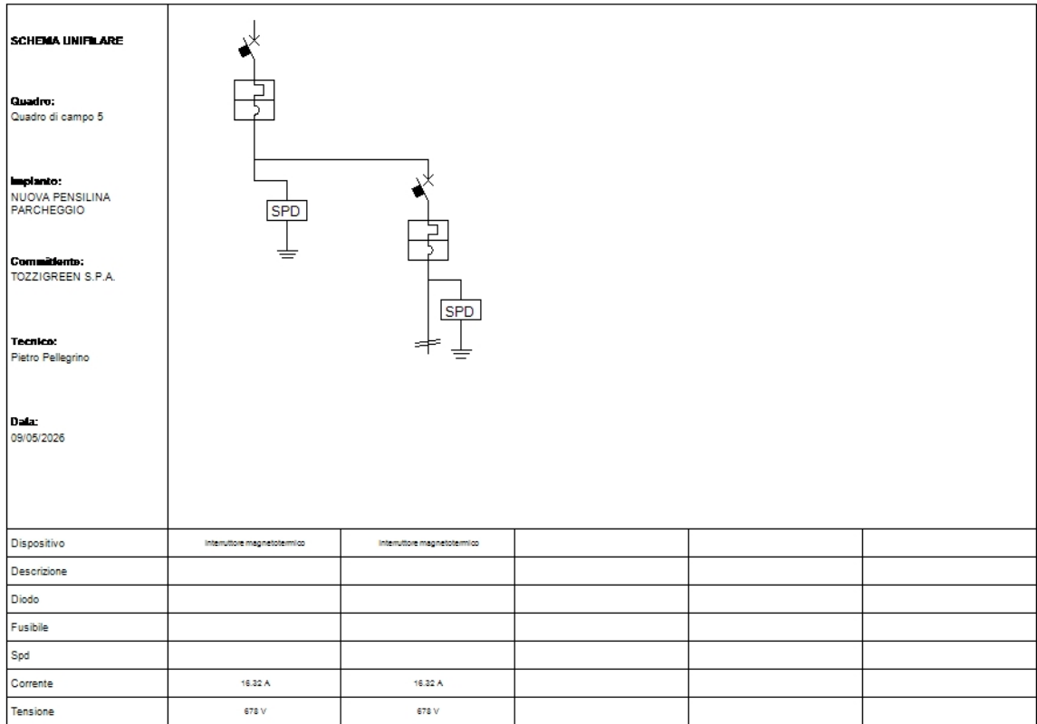
Fig. 11: Schema unifilare quadro "Quadro di campo 5"
