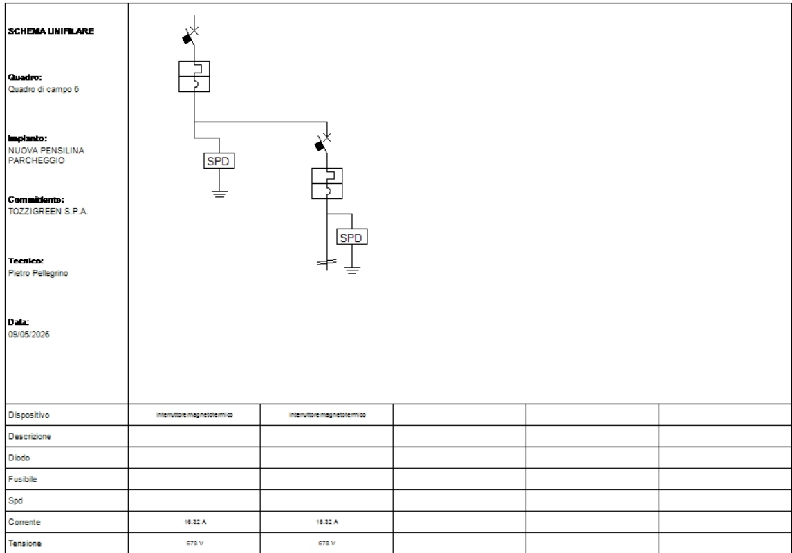
Fig. 12: Schema unifilare quadro "Quadro di campo 6"
