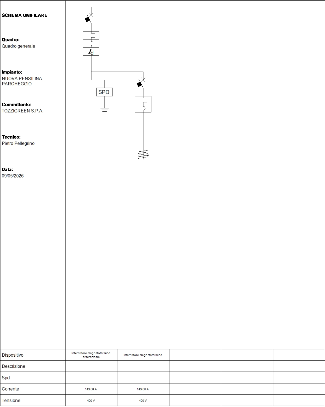
Fig. 5: Schema unifilare quadro "Quadro generale"
